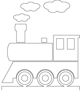
هَذَا قِطَارٌ
